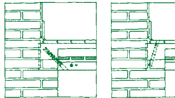
Deponering af Impel Bor-patrol i indmurede bjælker.
